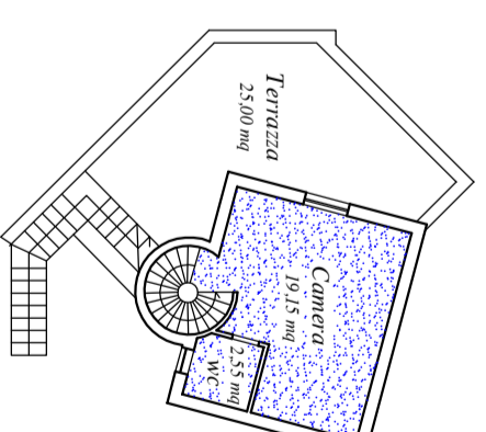
Piano Primo
